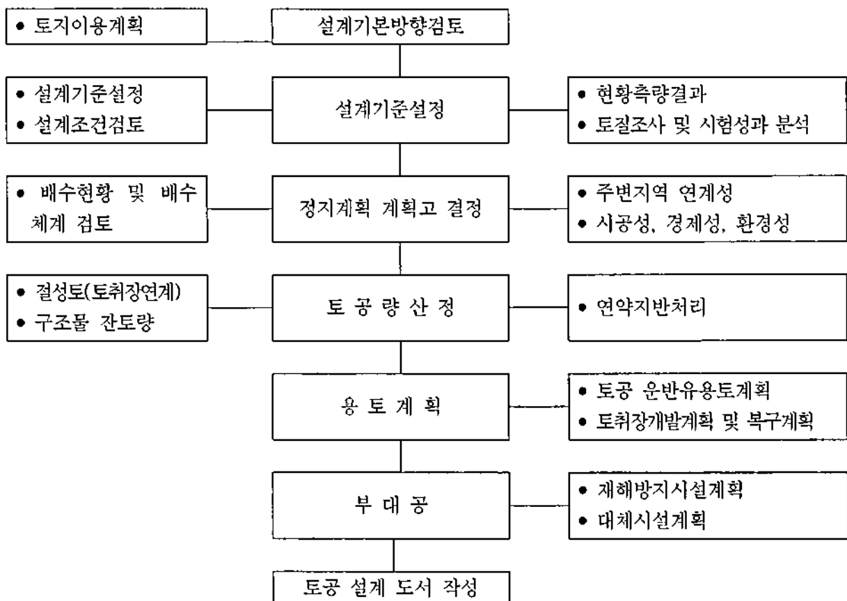
(그림 36) 부지정지 및 토공계획 흐름도
