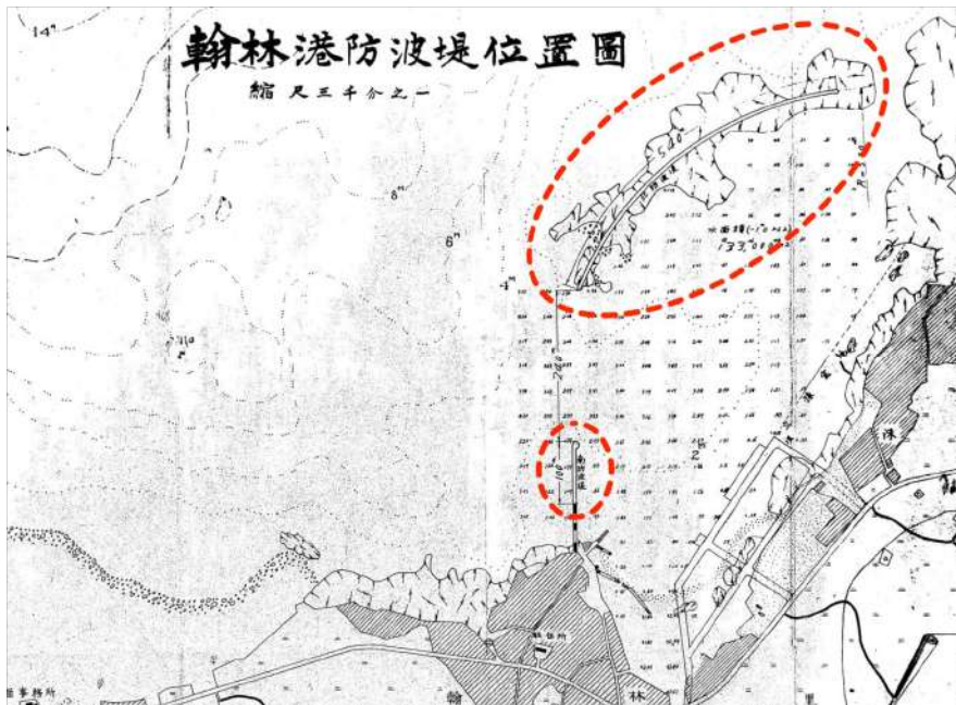
〈그림 2-4〉 한림항 2기 축항 방파제 위치도 75)
