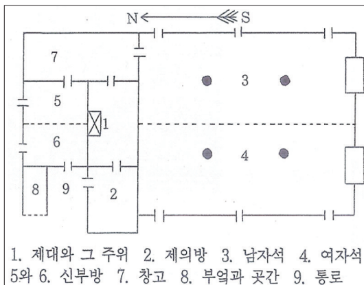
<그림 6> 김 스터왕 신부택 성당 평면
