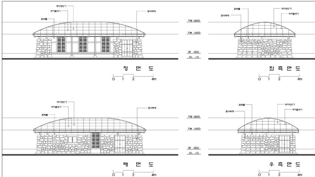
<그림 11> 사제관의 입면도
