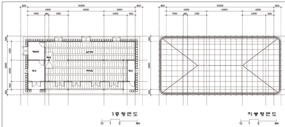
<그림 8> 하논성당의 평면도 및 지붕도
