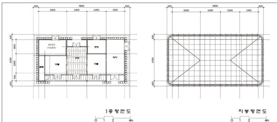
<그림 10> 사제관 평면도 및 지붕도
