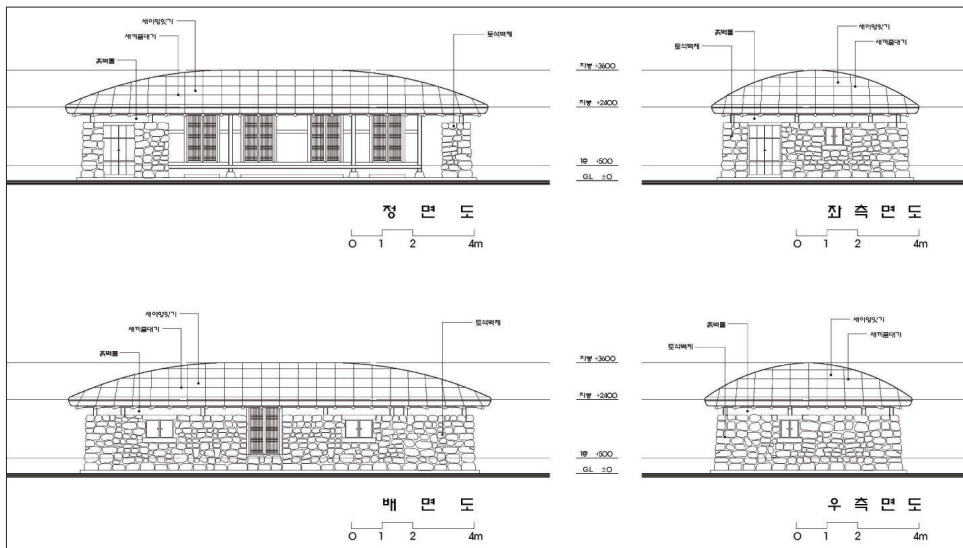
<그림 9> 하논성당의 입면도
