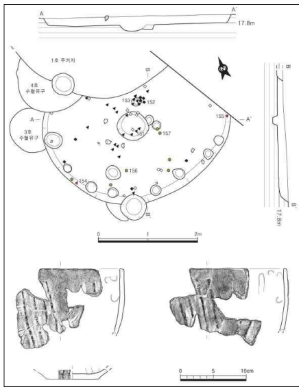
〈그림 11〉 I 구역 S3W1 Grid 2호주거지
