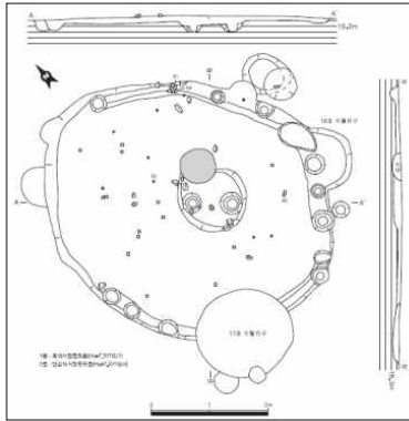
〈그림 3〉 I 구역 N4E1 Grid 1호주거지
