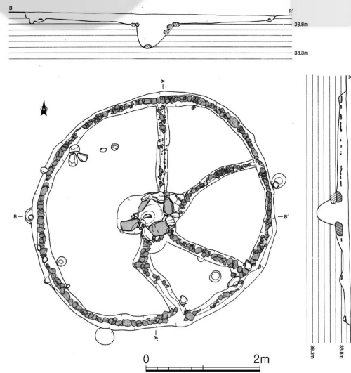
제주의도동유적 II-1구역 1호주거지 [도면 7] 벽구 주거지
