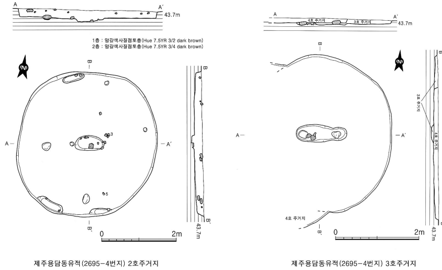
[도면 6] 무주공식 주거지(左)와 초석 주거지(右)
