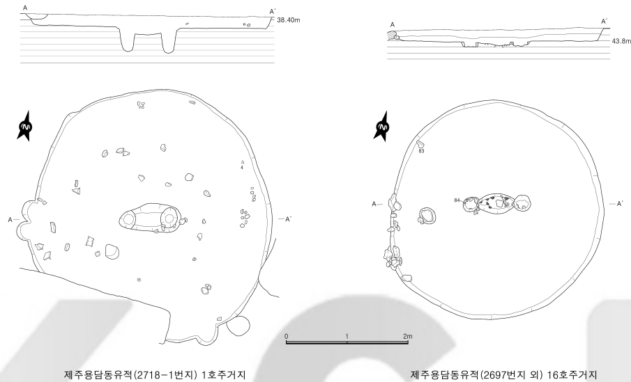
[도면 5] 깊은 주혈의 내주공식(左)과 얇은 주혈의 걸친주공식(右)
