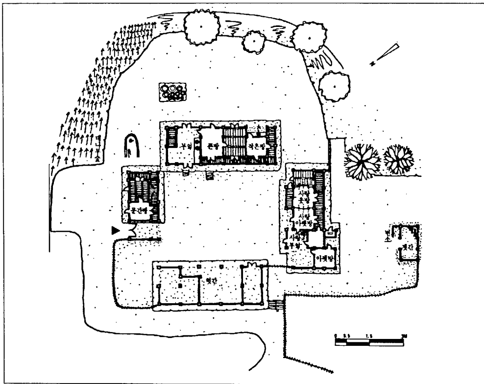
(圖 3-4-1) 영암 최성호 家 平面 및 配置圖17)
