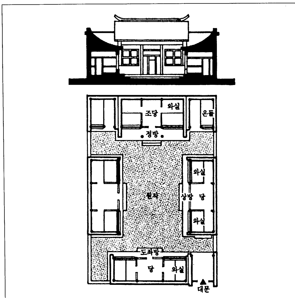
(圖 3-4-4) 中國 四合院의 傳統 民家 배치 및 斷面 (손세관, 1995, 80쪽)
