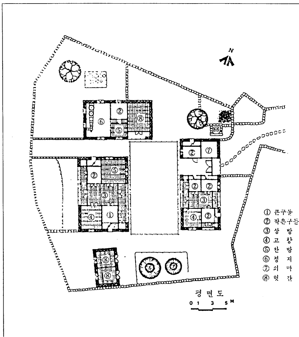
(圖 4-2-11) 新村里 曹氏 家 配置圖
