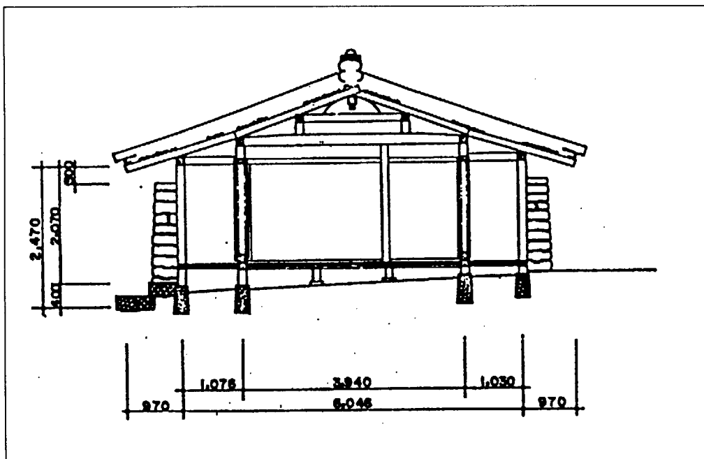
(圖 4-2-7) 안거리 斷面圖
