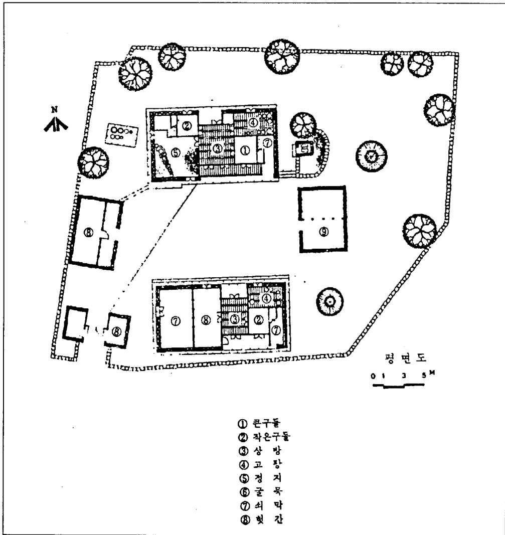
(圖 4-2-9) 城邑里 曹氏 家 配置圖
