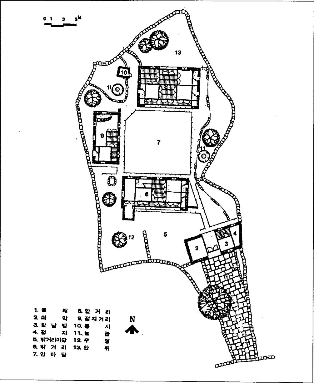
(圖 4-2-5) 金氏 家 配置圖
