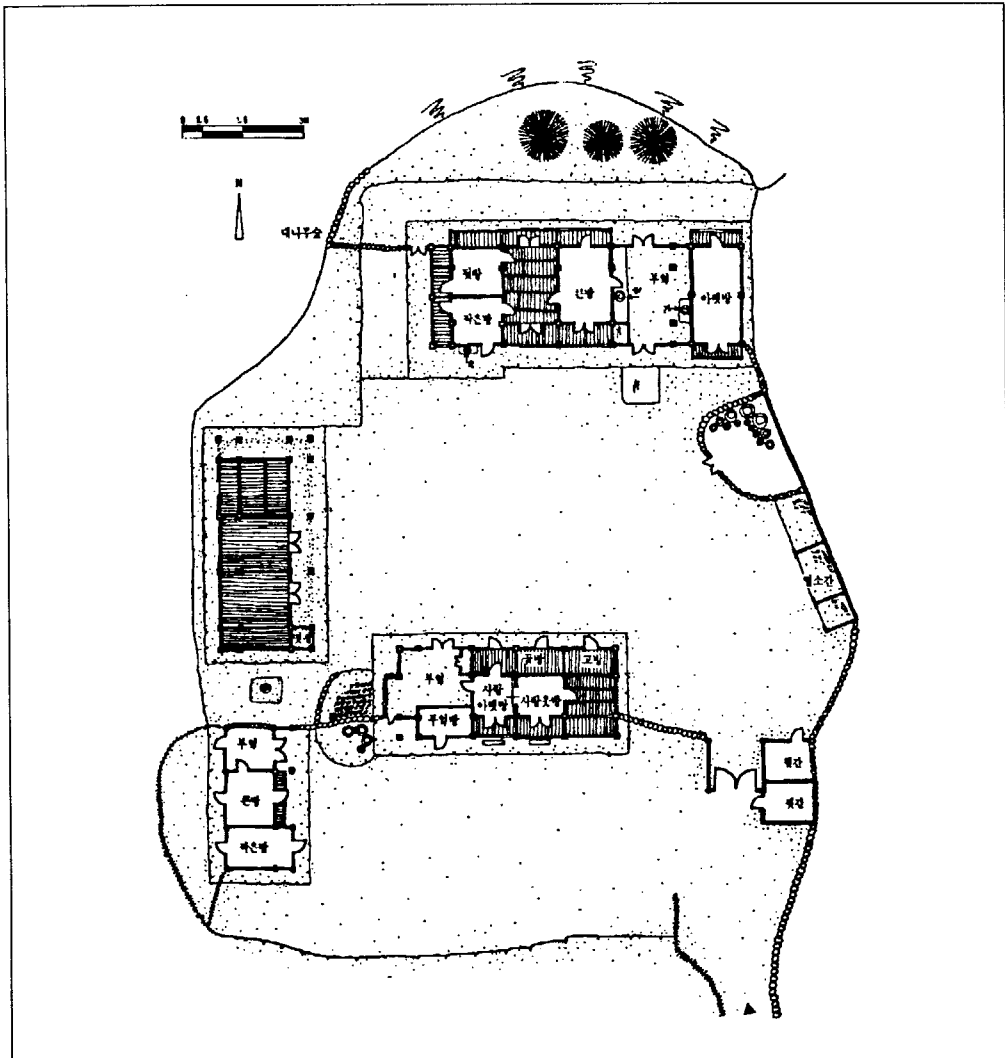
(圖 3-4-2) 보성군 득량면 이식래 家 平面 및 配置圖 18)
