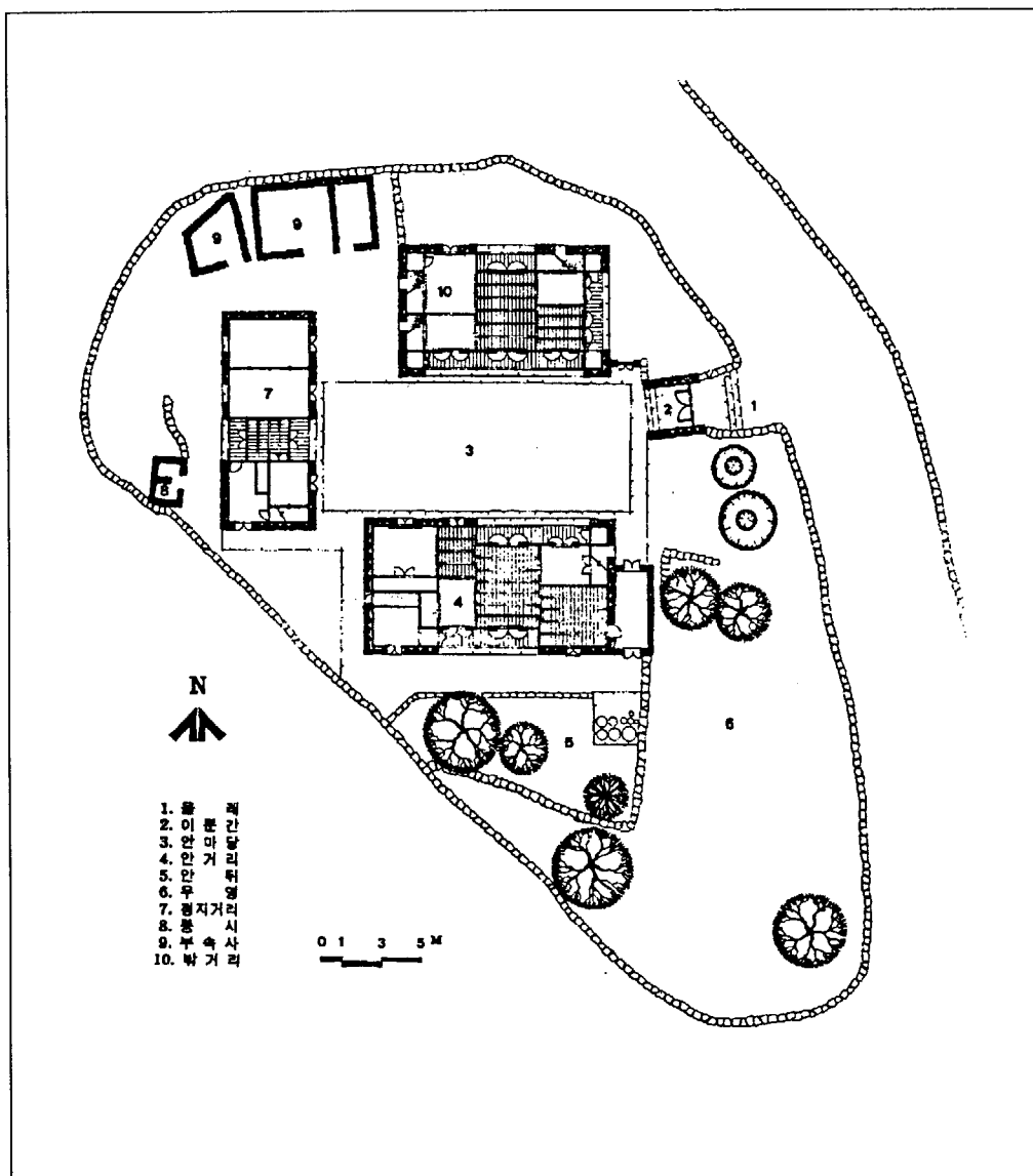
(圖 4-2-13) 朝天里 黃氏 家 配置圖
