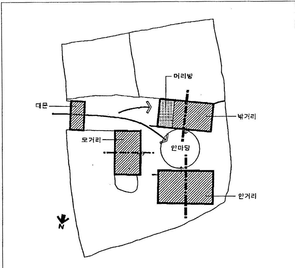
(圖 4-2-16) 外部空間의 構成
