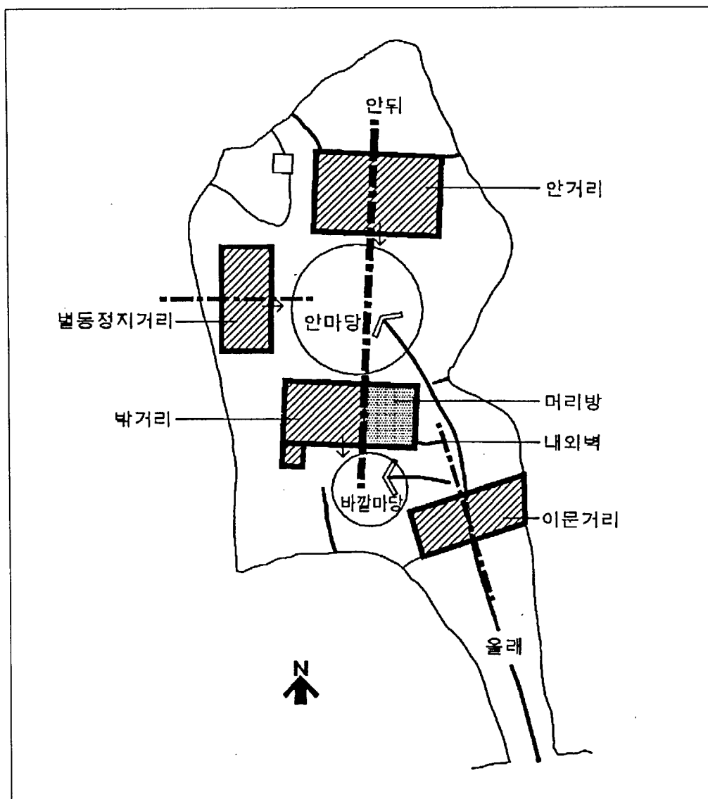
(圖 4-2-6) 外部空間의 構成
