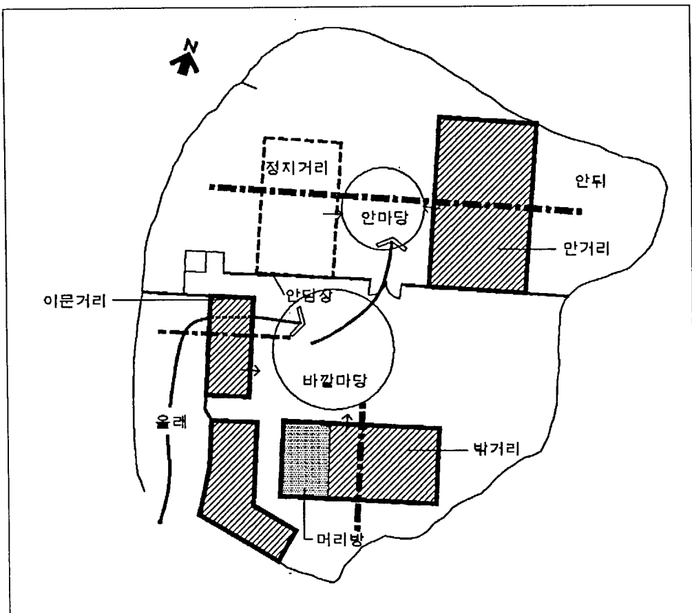
(圖 4-2-2) 外部空間의 構成
