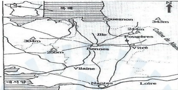
<그림 13> Saint-Christophes-des-Bois 지역 43)
