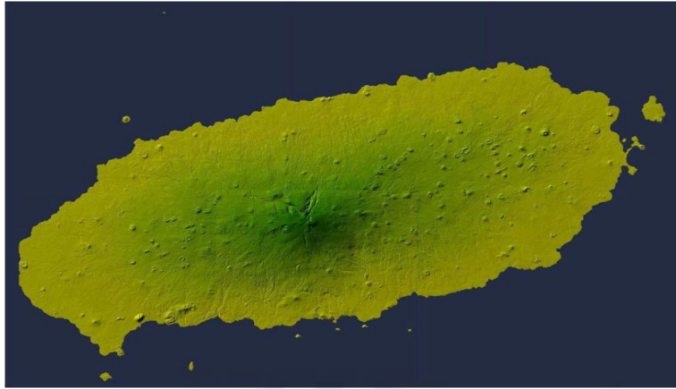
〈그림 3〉 지표기복이 없는 제주도의 모습
