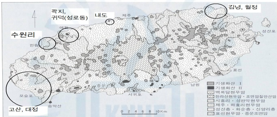
<그림 4> 제주도의 지질 38)
